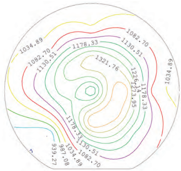
Abb. 2: Mapping der Elektronenmobilität \mu eines 4-Inch-Wafers mit einer AlScN-HEMT-Struktur, durchschnittliche Elektronenmobilität: 1203 cm 2 /Vs
